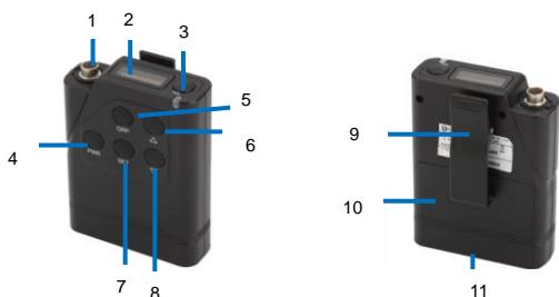
LTWI-BP750, 벨트팩 전면과 후면 패널 상세
