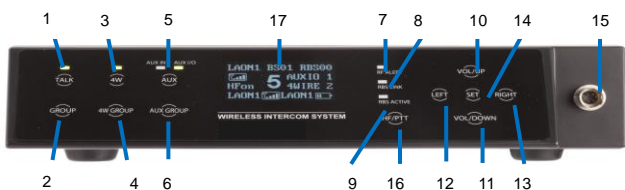
LTWI-BS750, 베이스 스테이션 전면 패널 상세
