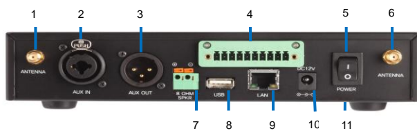
LTWI-BS750, 베이스 스테이션 후면 패널 상세
