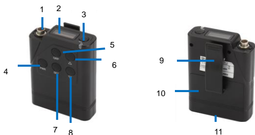
LTWI-BP550, 벨트팩 전면과 후면 패널 상세
