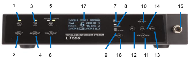
LTWI-BS550, 베이스 스테이션 전면 패널 상세
