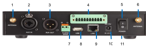
LTWI-BS550, 베이스 스테이션 후면 패널 상세
